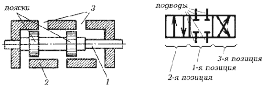
Рис.3.1. Схема (а) и обозначение (б) гидрораспределителя
