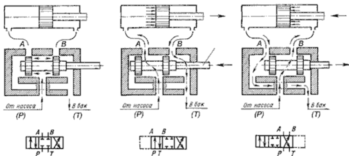
Рис.3.2. Схема работы золотникового гидрораспределителя
